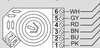
Переключатель режимов
