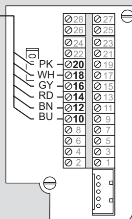
Блок управления
